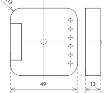
MINI
