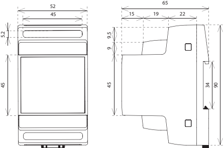
3-MODUL
