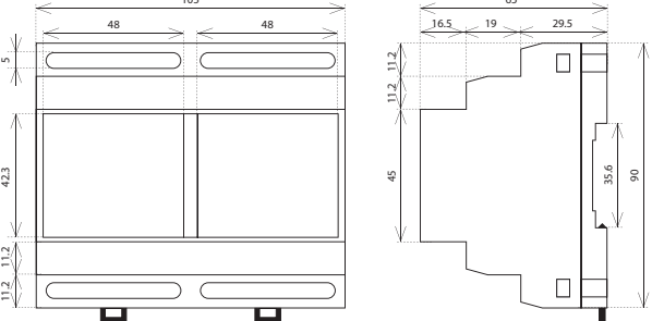
6-MODUL
