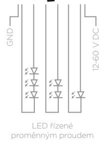
LED řízené proměnným proudem
